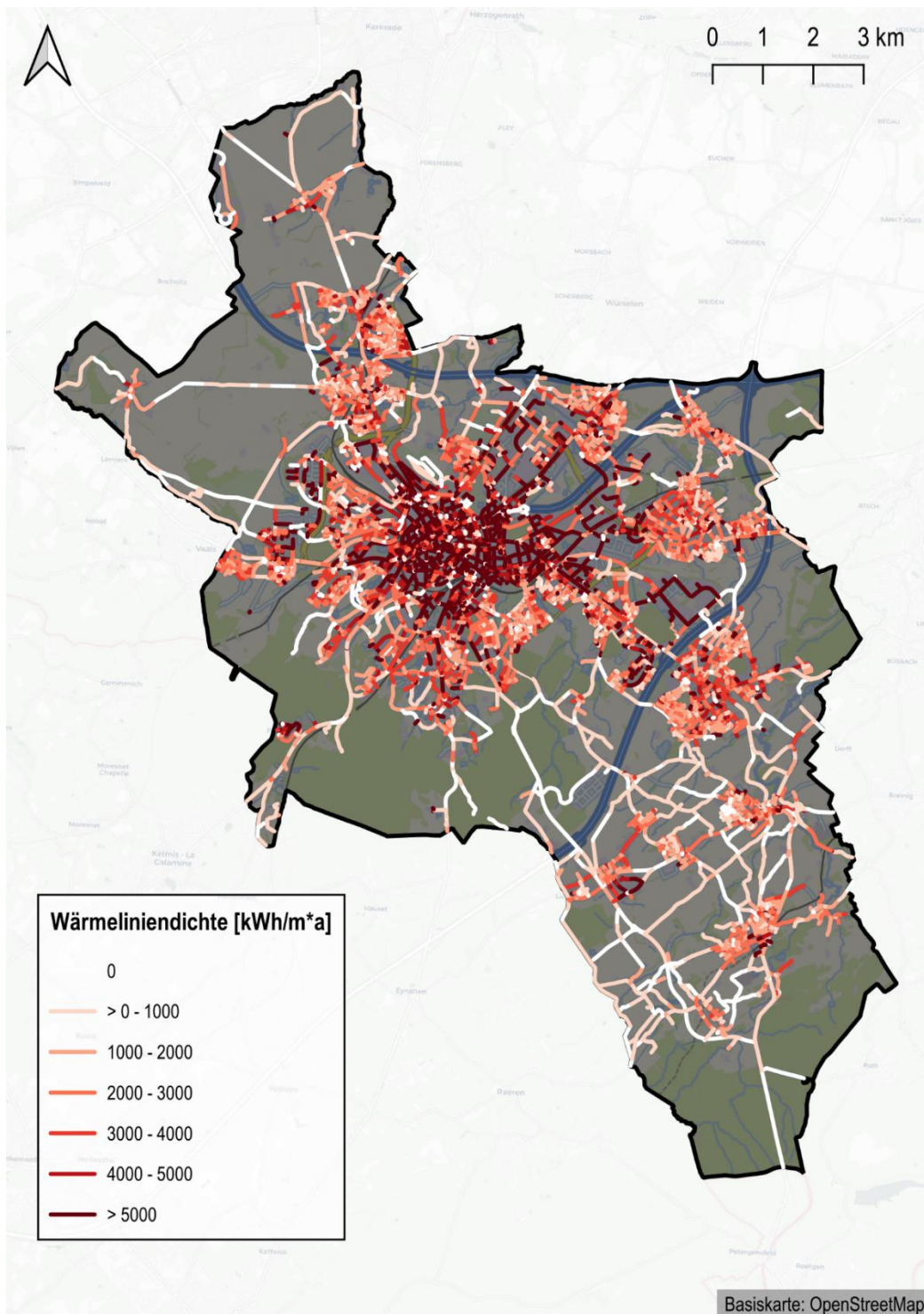
Abbildung 30: Wärmelinienendichte
