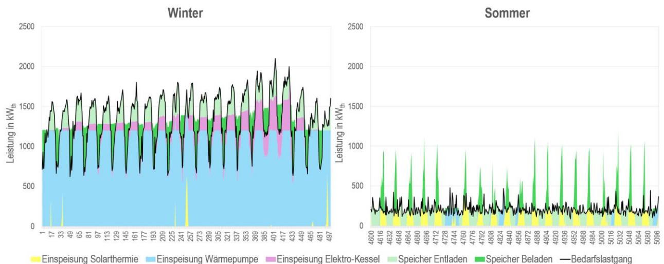
Abbildung 81: Lastgänge des Wärmebedarfs und der Wärmeerzeugung für das Nahwärmekonzept in Kornelimünster. Links: Winter, rechts: Sommer
