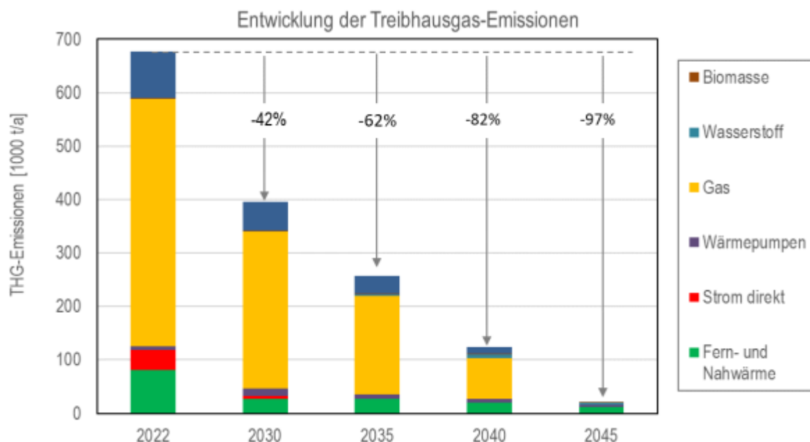
Abbildung: Treibhausgas-Emissionen in der Wärmeversorgung im Zeitverlauf bis 2045
