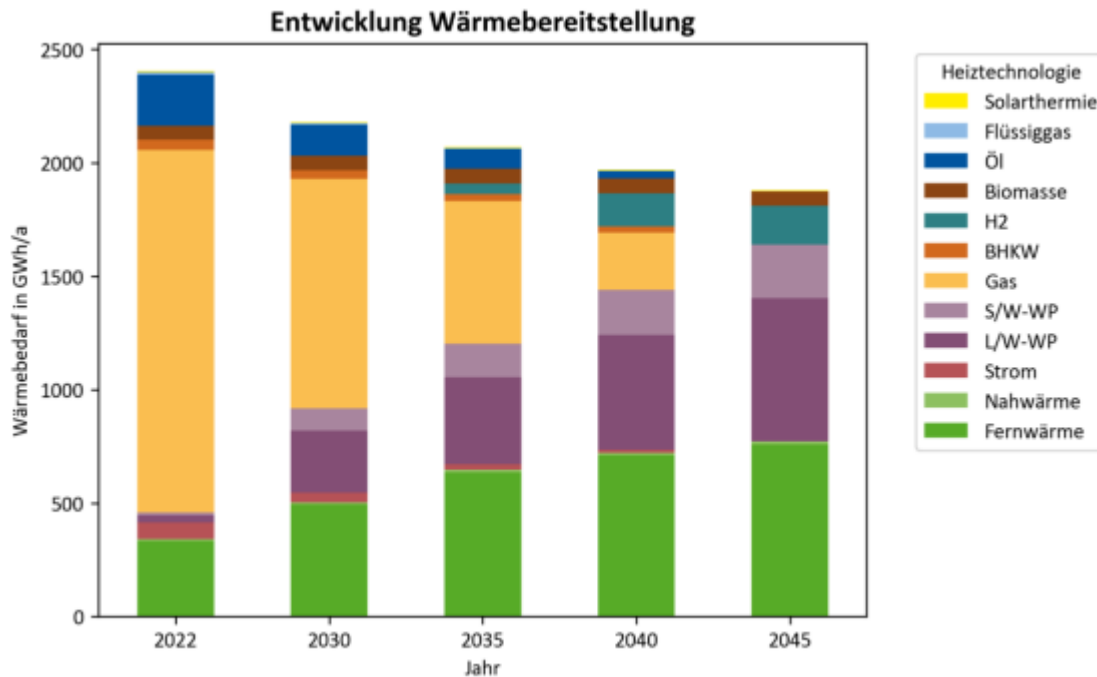
Abbildung: Wärmebedarfsdeckung im Zeitverlauf bis 2045
