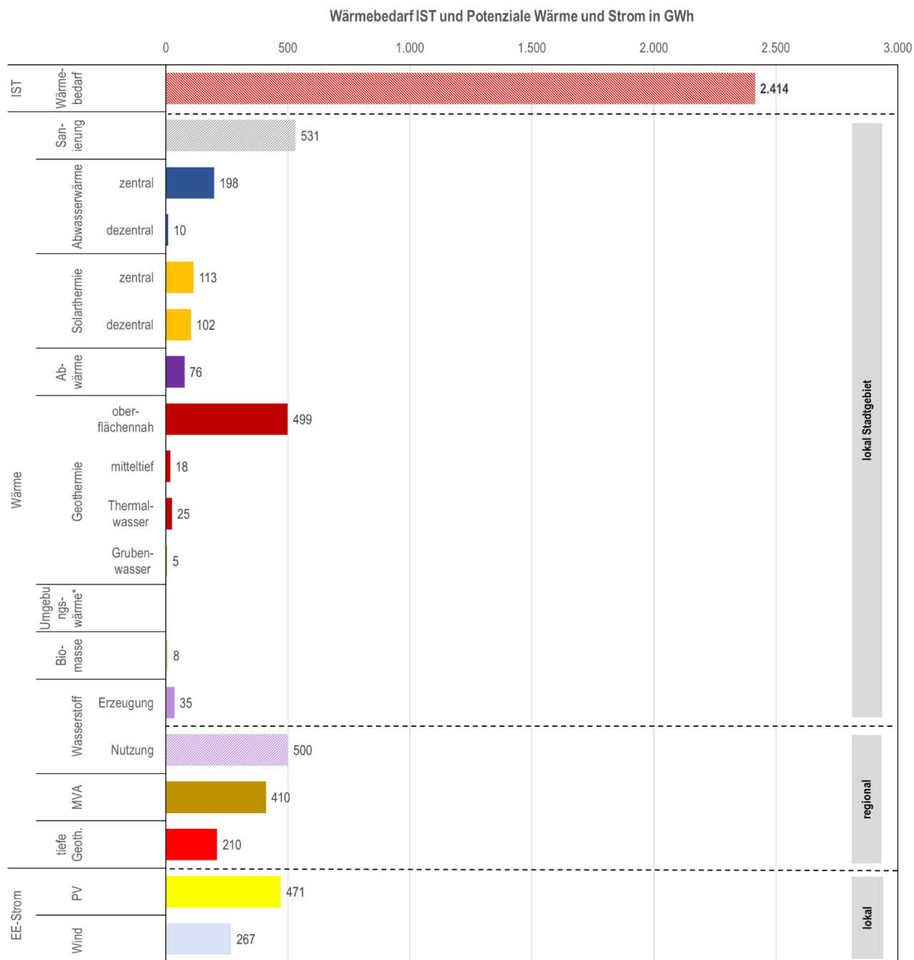
Abbildung 66: Zusammenfassung der technisch nutzbaren Potenziale
