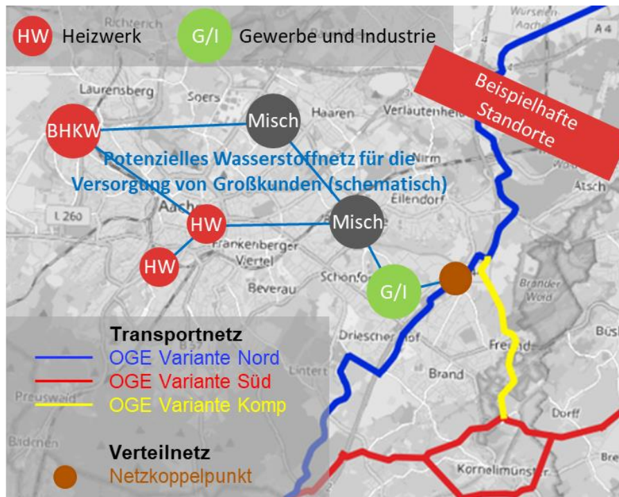
Abbildung 94: schematische Darstellung eines H 2 -Verteilnetzes in Aachen
