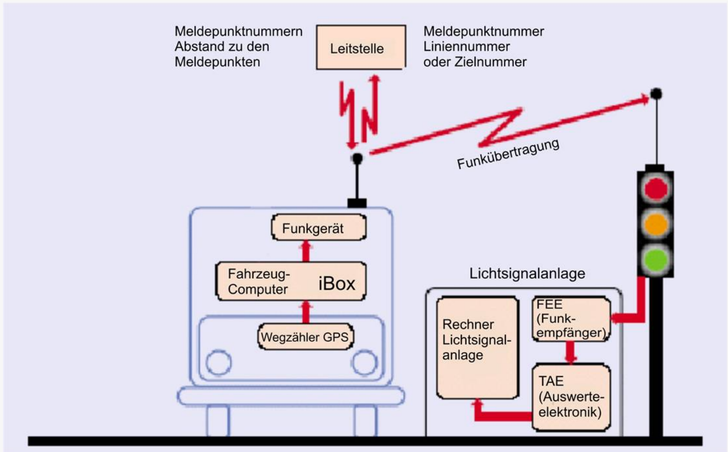
Das Schaubild zeigt die wichtigsten Komponenten des RBL im Zusammenspiel mit der Vorrangschaltung an Lichtzeichenanlagen.
