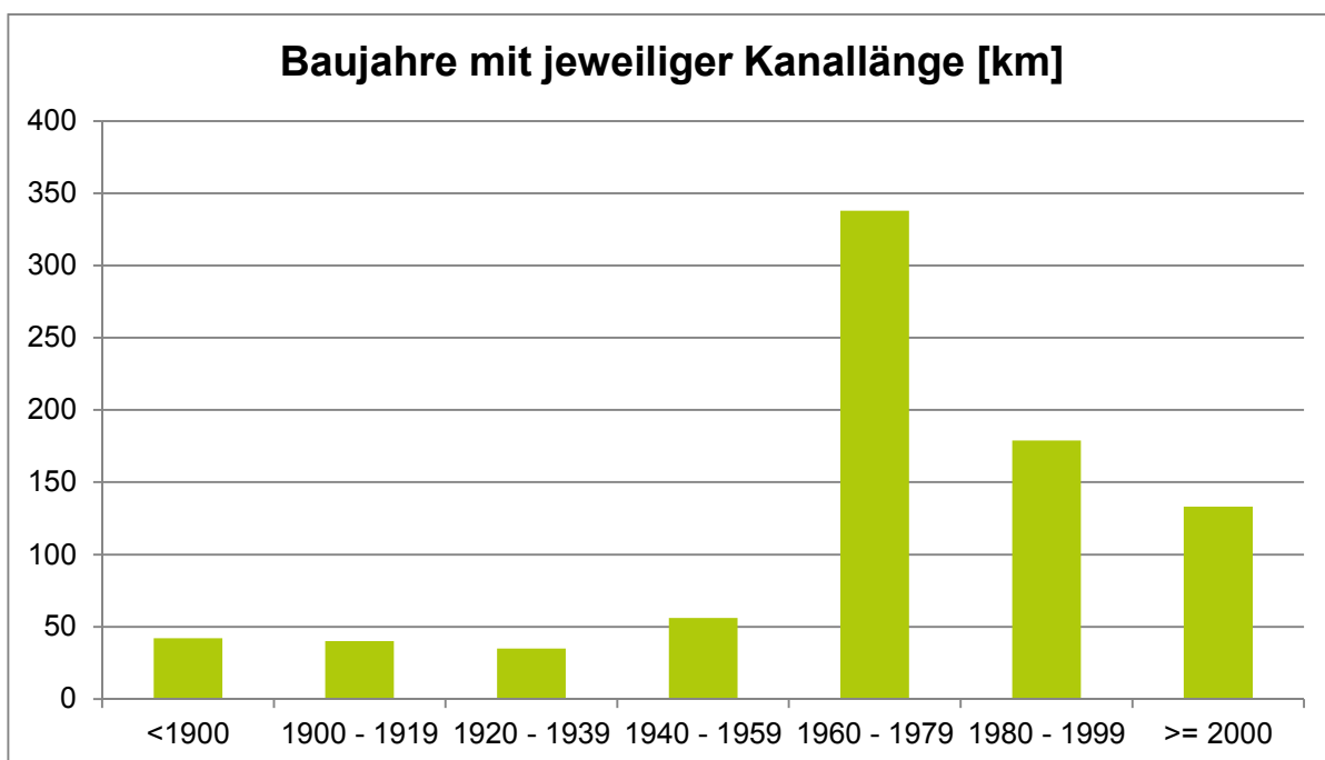
Abbildung 1: Altersstruktur des Aachener Kanalnetzes (2018)
