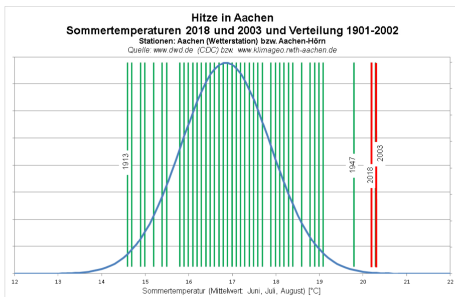
Abb. 7: Hitze in Aachen – Sommertemperaturen 2018 und 2003 sowie die Verteilung der Sommertemperaturen für die Jahre 1901 – 2002 mit den bis 2002 kältesten und wärmsten Sommern (1913 und 1947), darin verzeichnet 2003 und 2018
