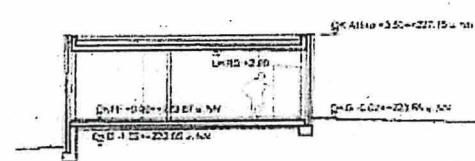
Umkleiden - Querschnitt
