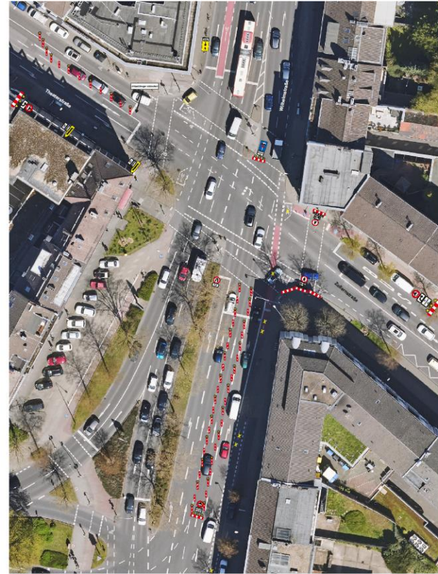
Verkehrszeichenplan Sperrung Wilhelmstraße Anlage 4 - Normstraße / Theaterstraße / Zücherstraße
