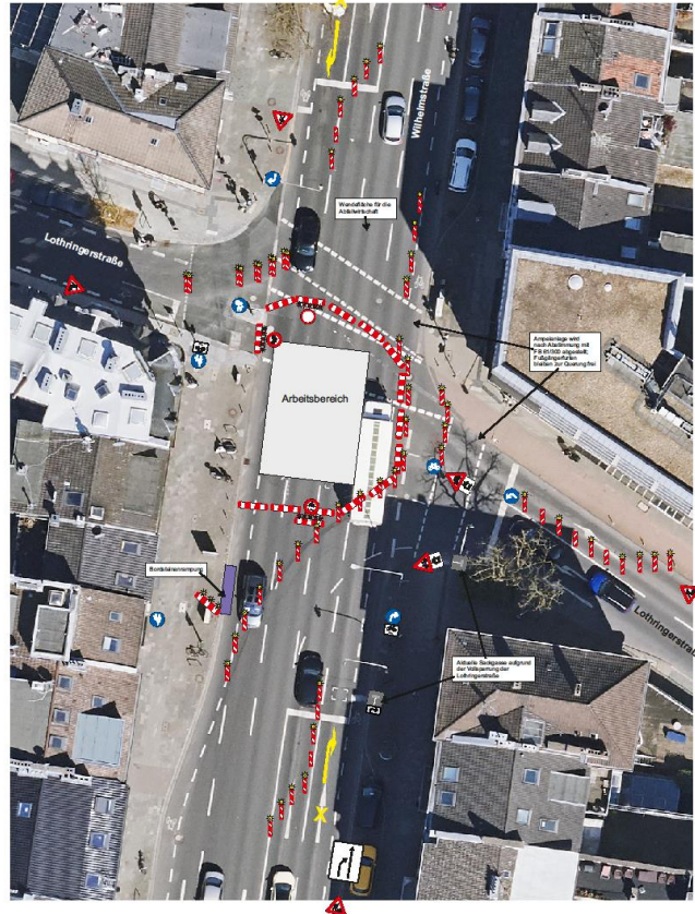
Verkehrszeichenplan Sperrung Wilhelmstraße Anlage 1 - Wilhelmstraße / Lothringstraße
