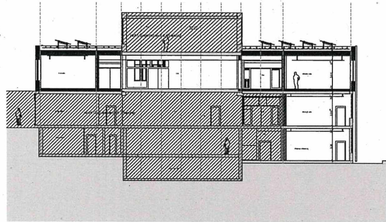
Schnitt AA
