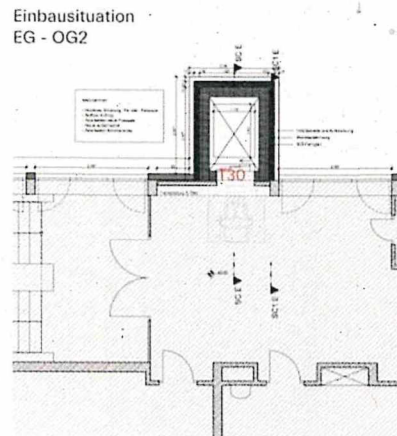
Einbausituation UG
