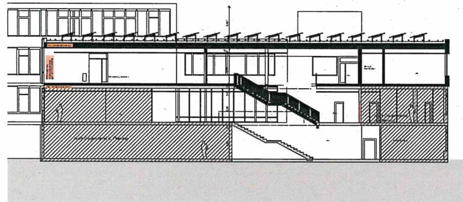
Schnitt BB
