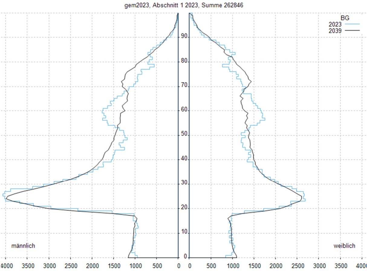
Abb. 7: Vergleich der Alterspyramide 2023 mit der Medium-Variante 2039
