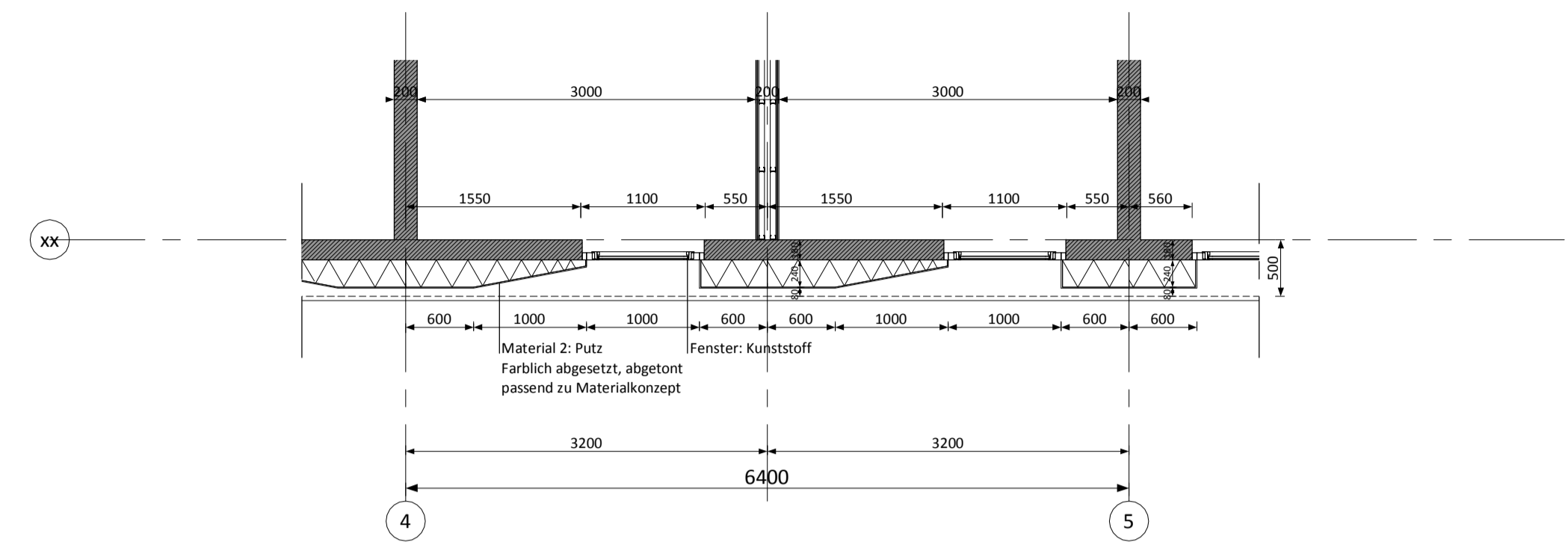
Schnitt H1
