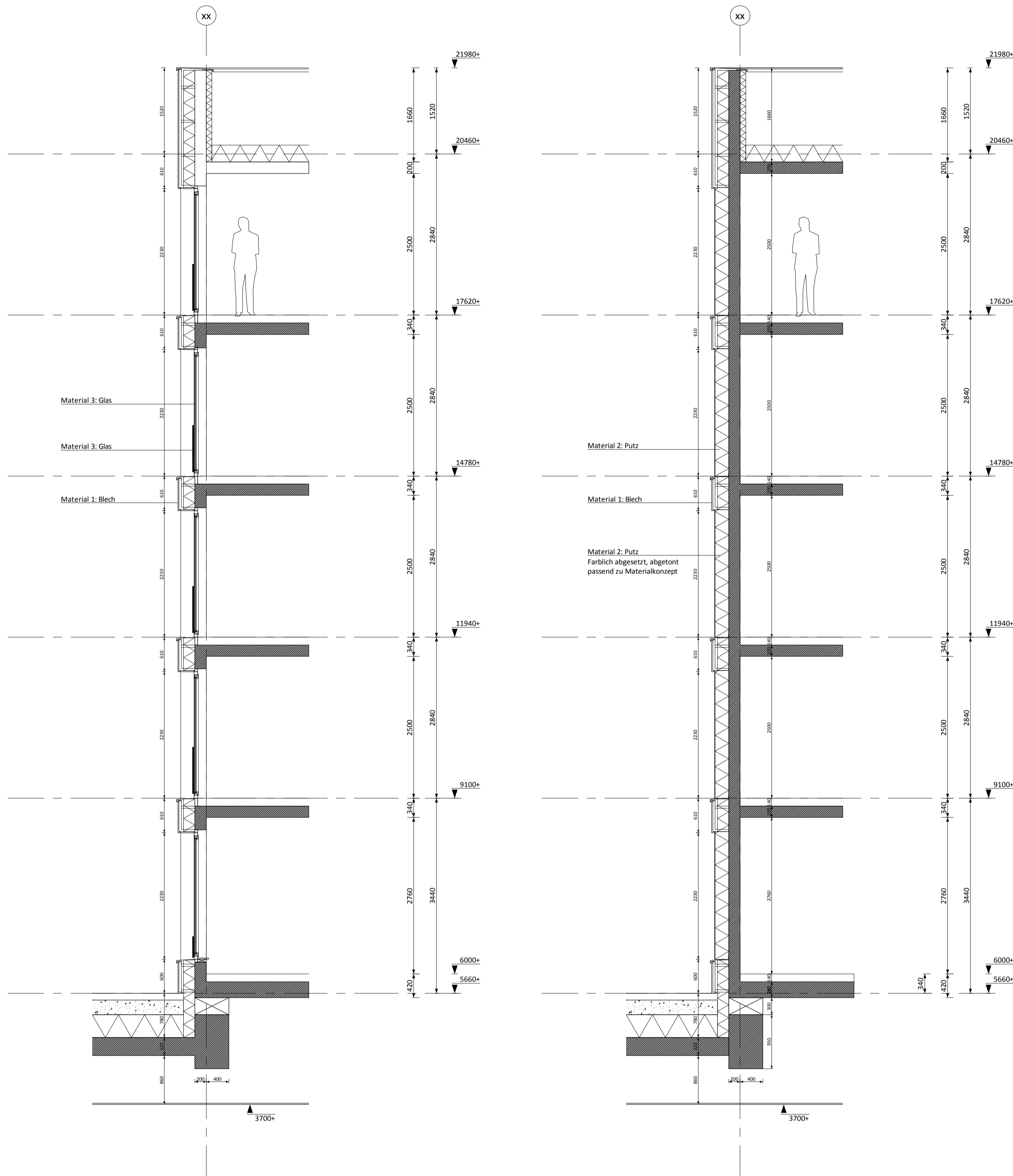
Schnitt V1
