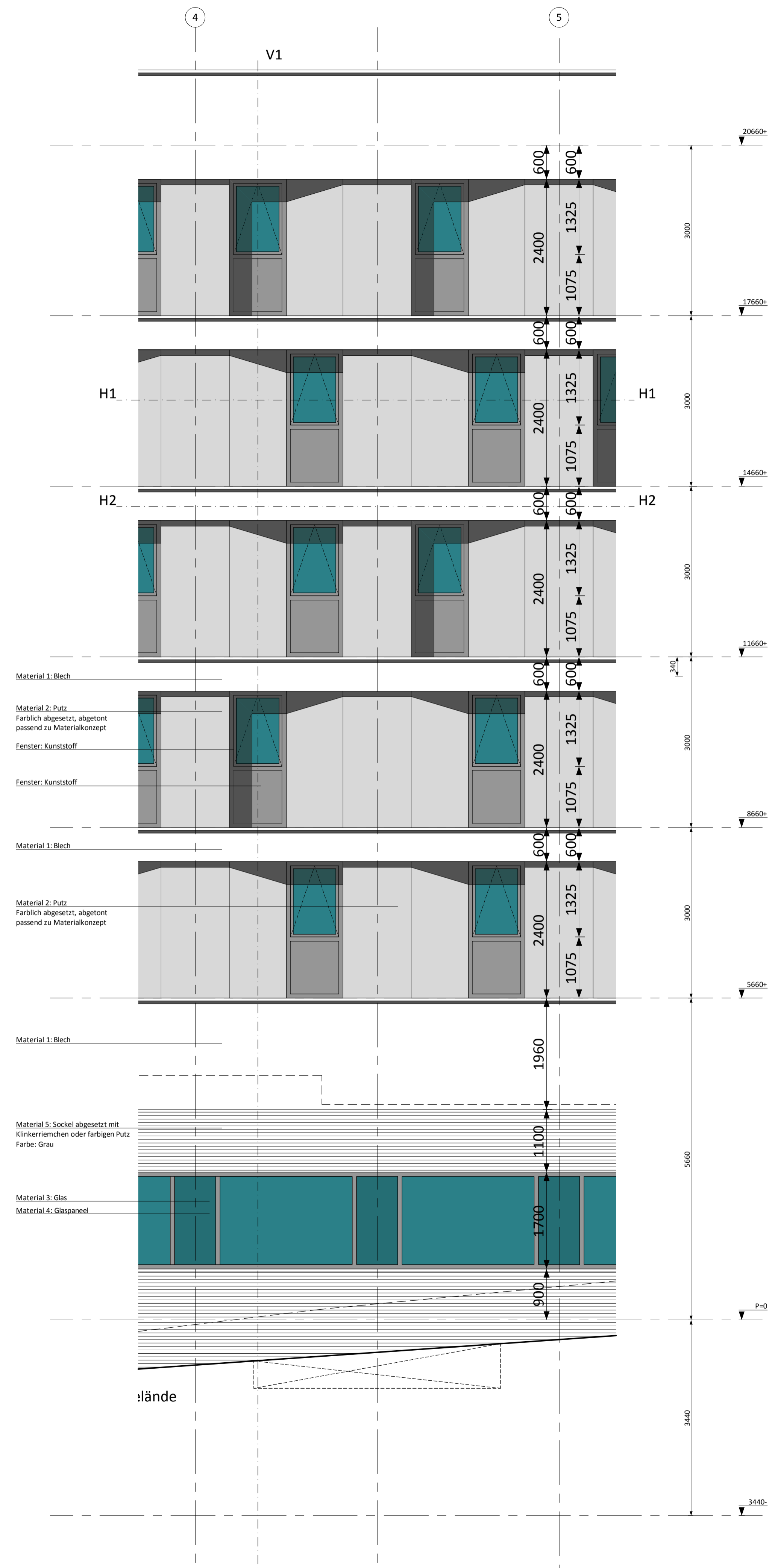
Fassade Hotel
