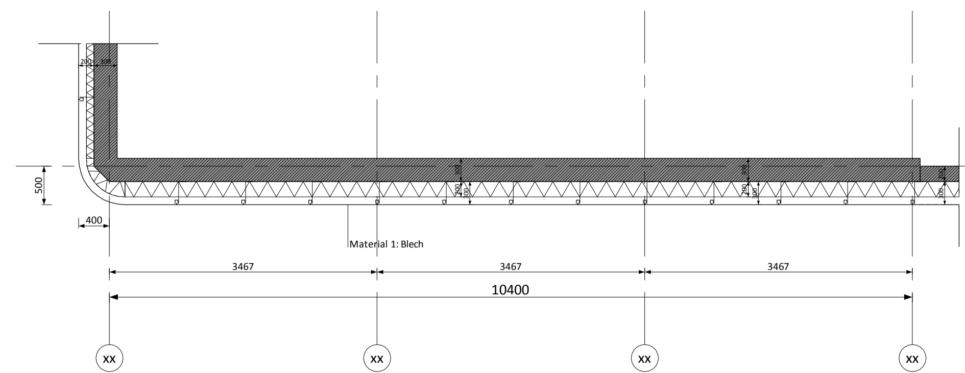
Schnitt H2 (Stirnseite)
