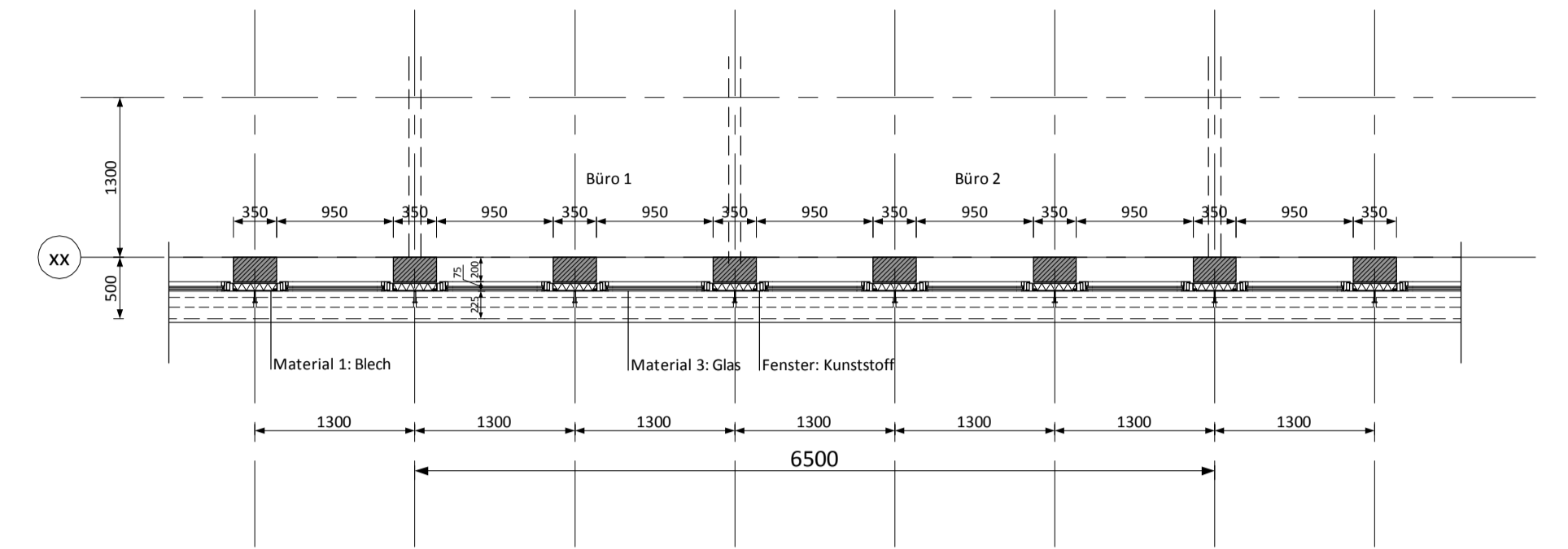
Schnitt H1
