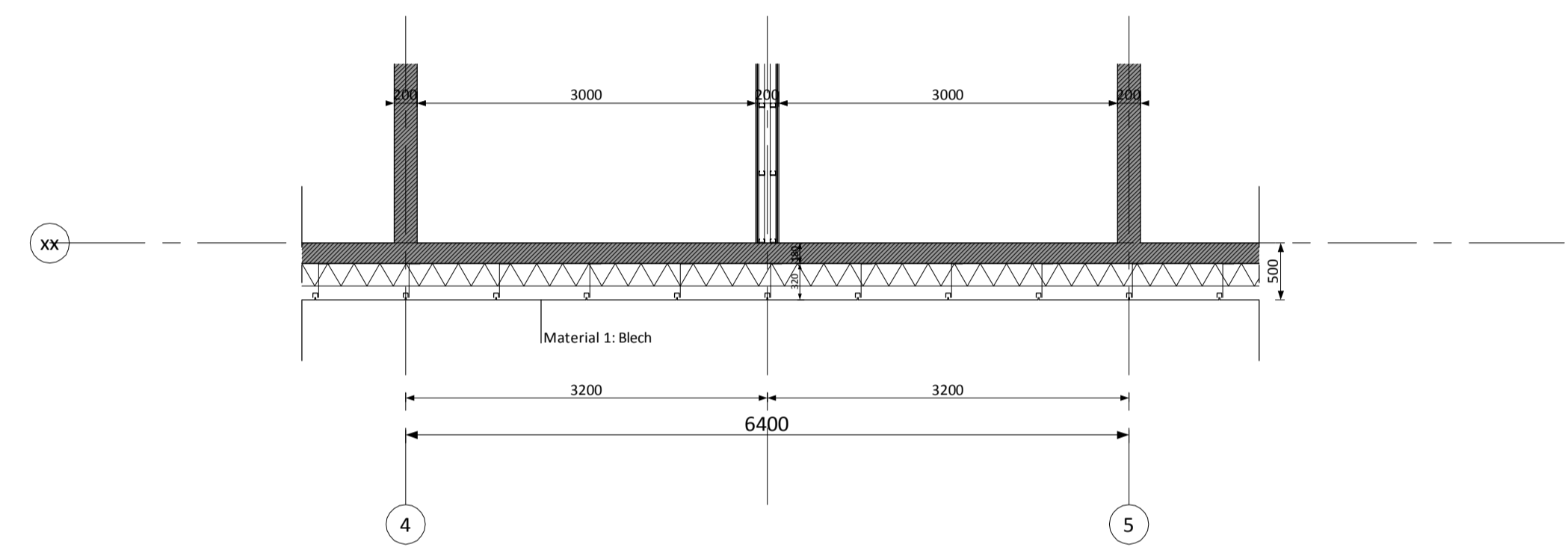
Schnitt H2
