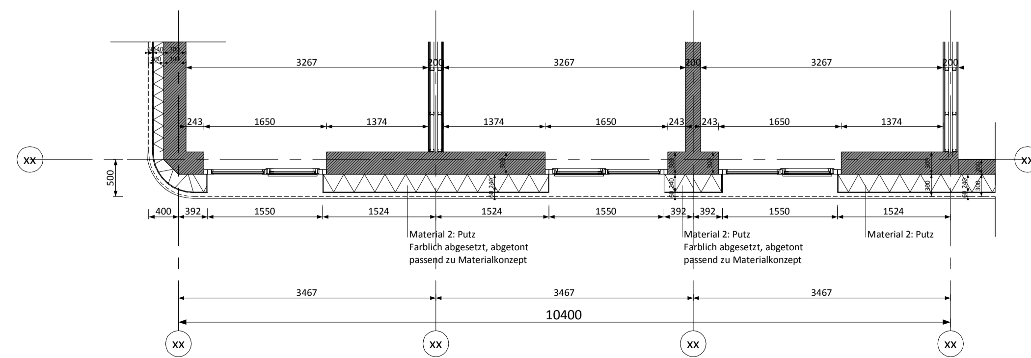
Schnitt H1 (Stirnseite)
