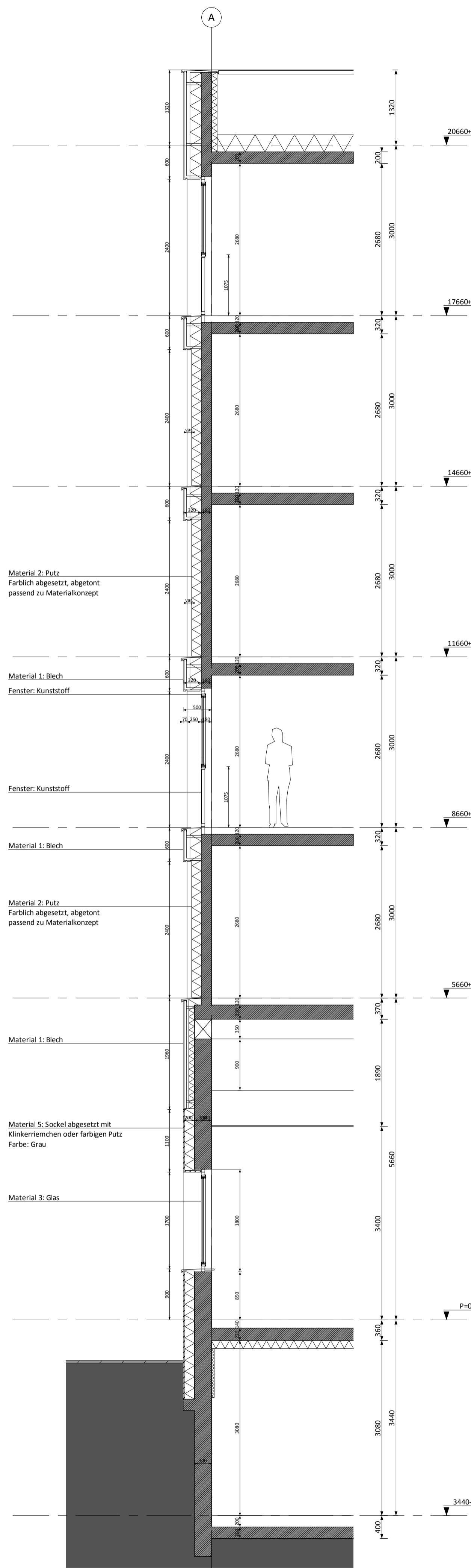
Schnitt V1
