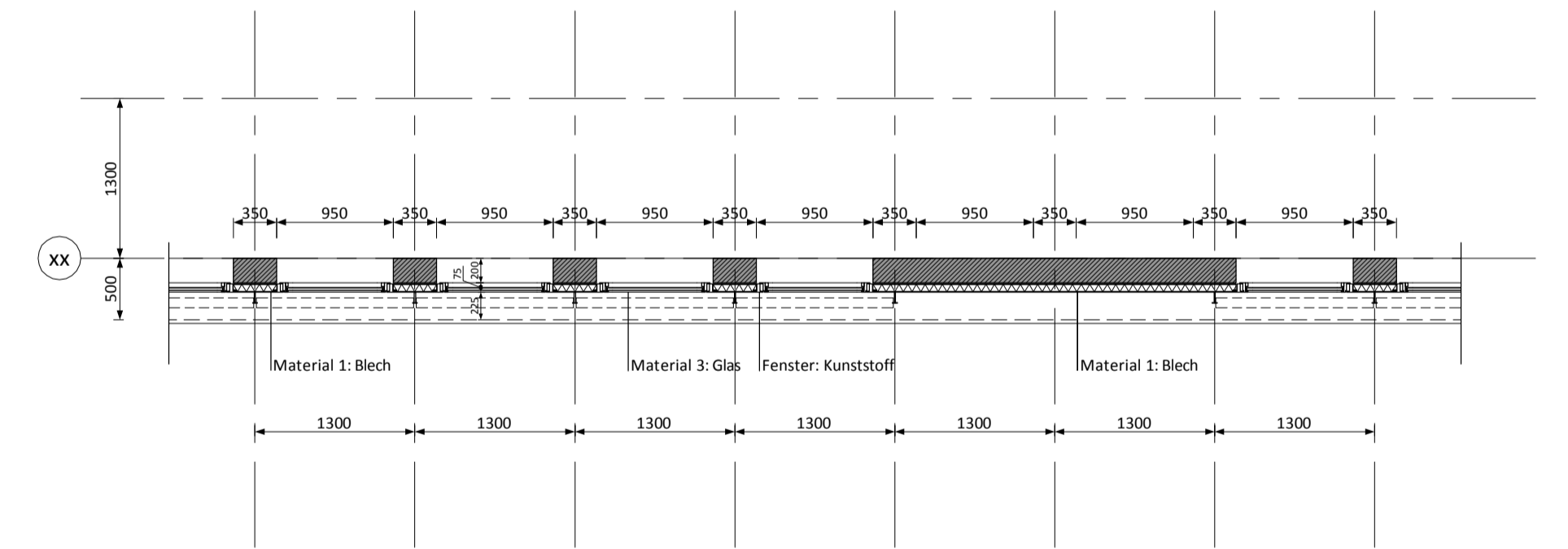
Schnitt H3
