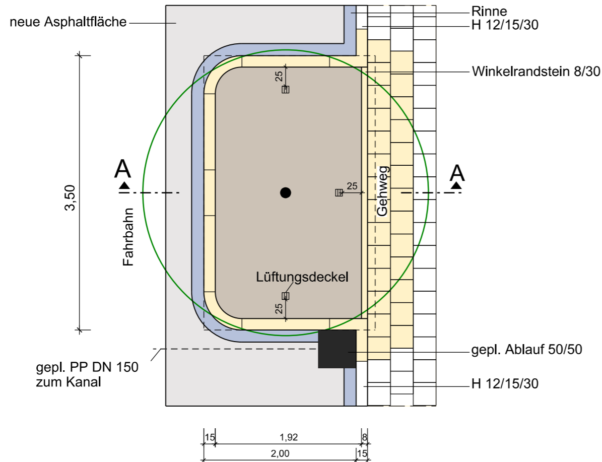
Draufsicht
