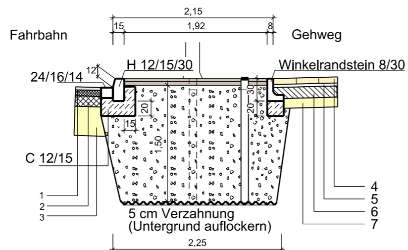
Schnitt A-A
