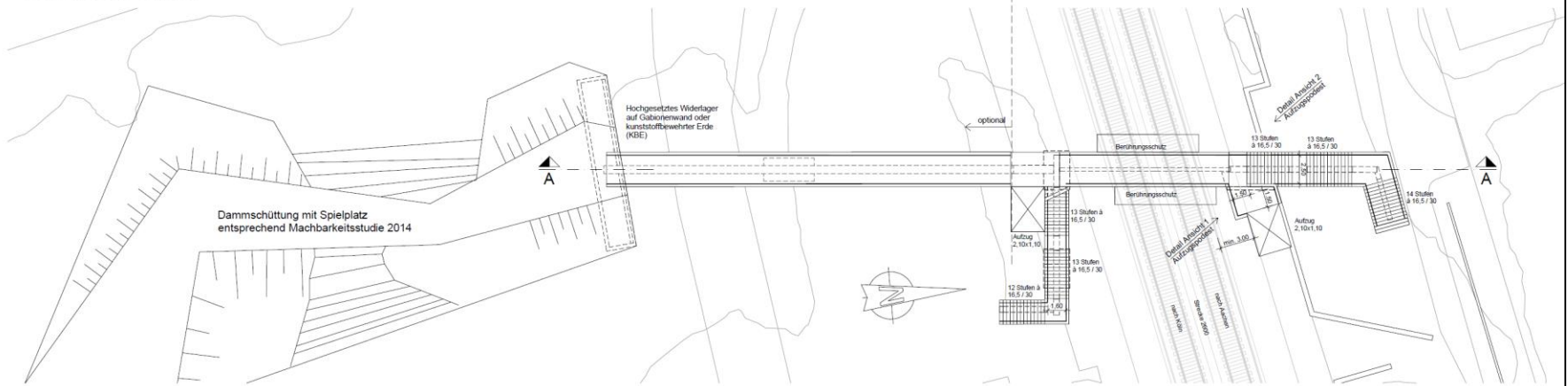
Draufsicht M 1:200
