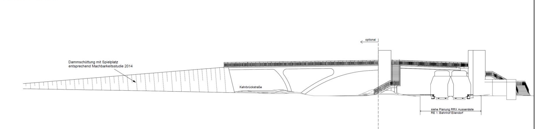
Ansicht M 1:200
