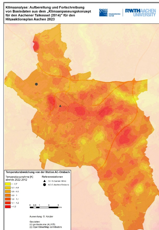
Abbildung 3: Modellierte Temperaturveränderungen in Aachen von 2012-2022 für die Abendstunden.
