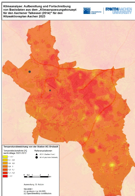
Abbildung 2: Modellierte Temperaturveränderungen in Aachen von 2012-2022 für die Nachmittagsstunden.
